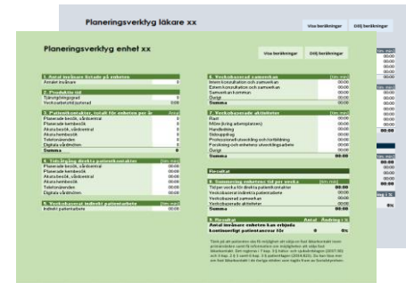
Planeringsverktyg
